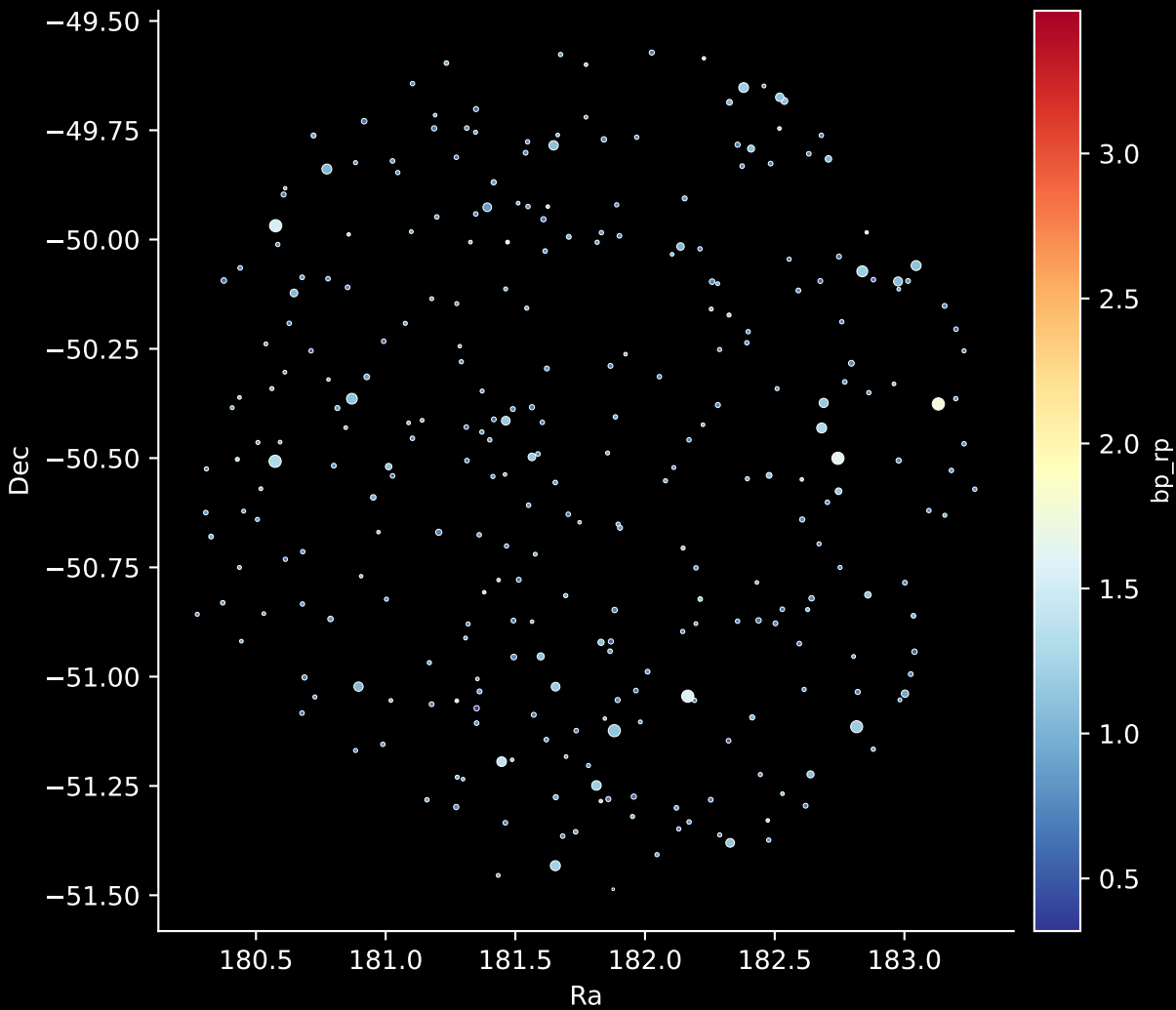
GALAH DR4 Field: [608] Stars: 300
