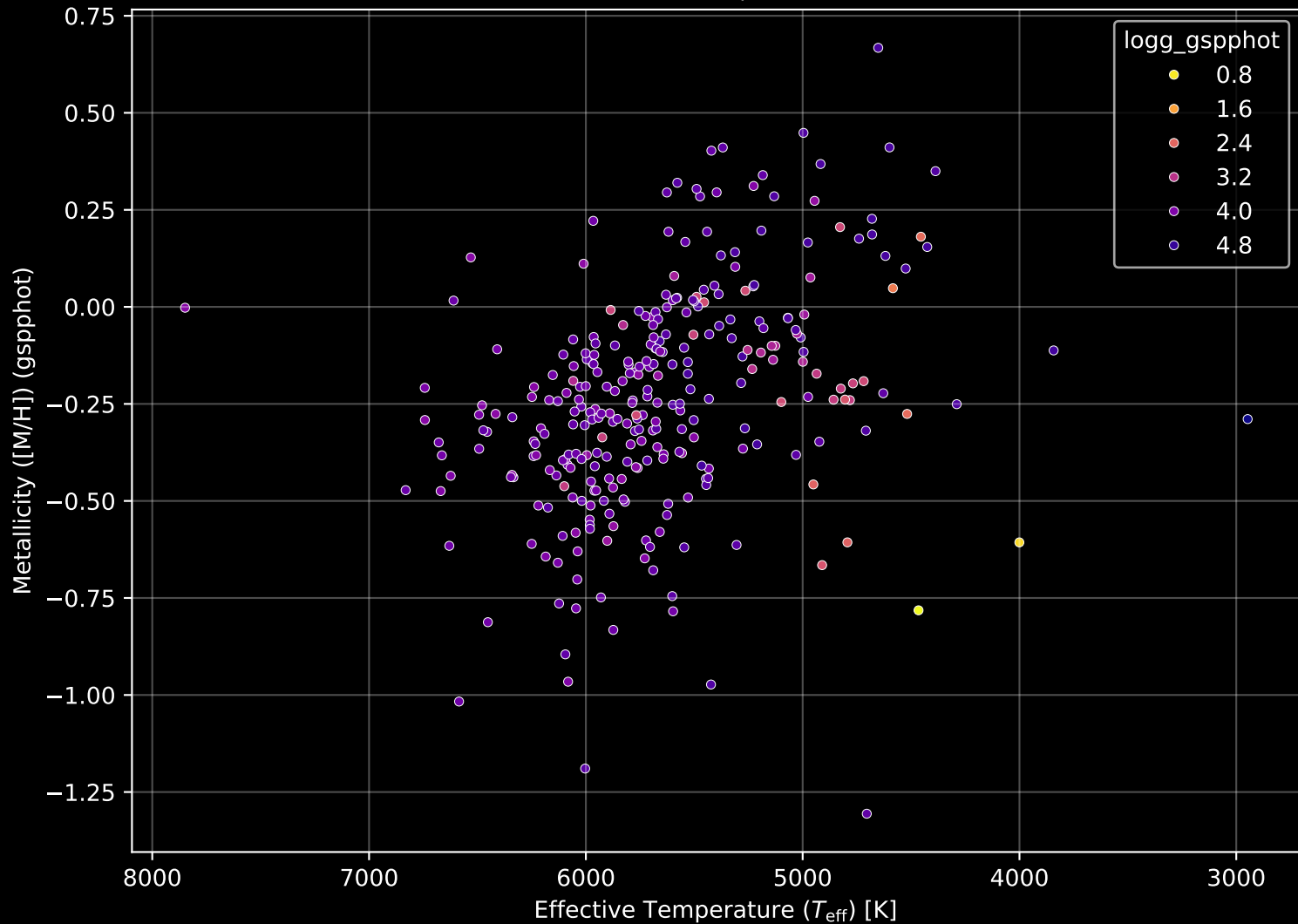
GALAH DR4 Field: [608] Stellar Population Parameters (n= 300)
