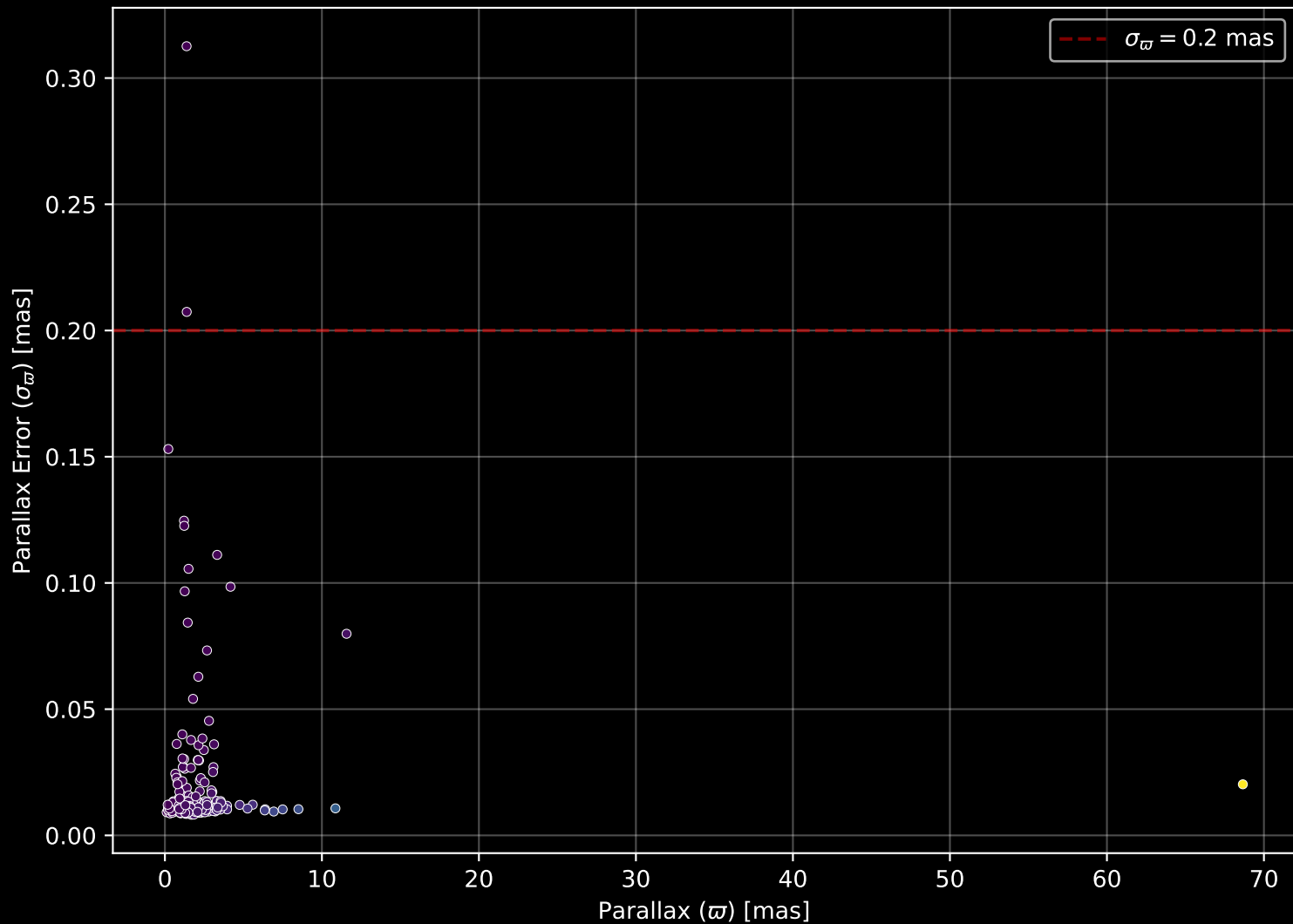
GALAH DR4 Field: [608] Parallax Quality (n= 300)
